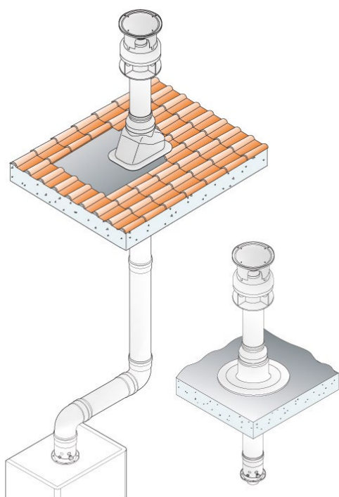
Коаксиальная система (60/100, 80/125)
